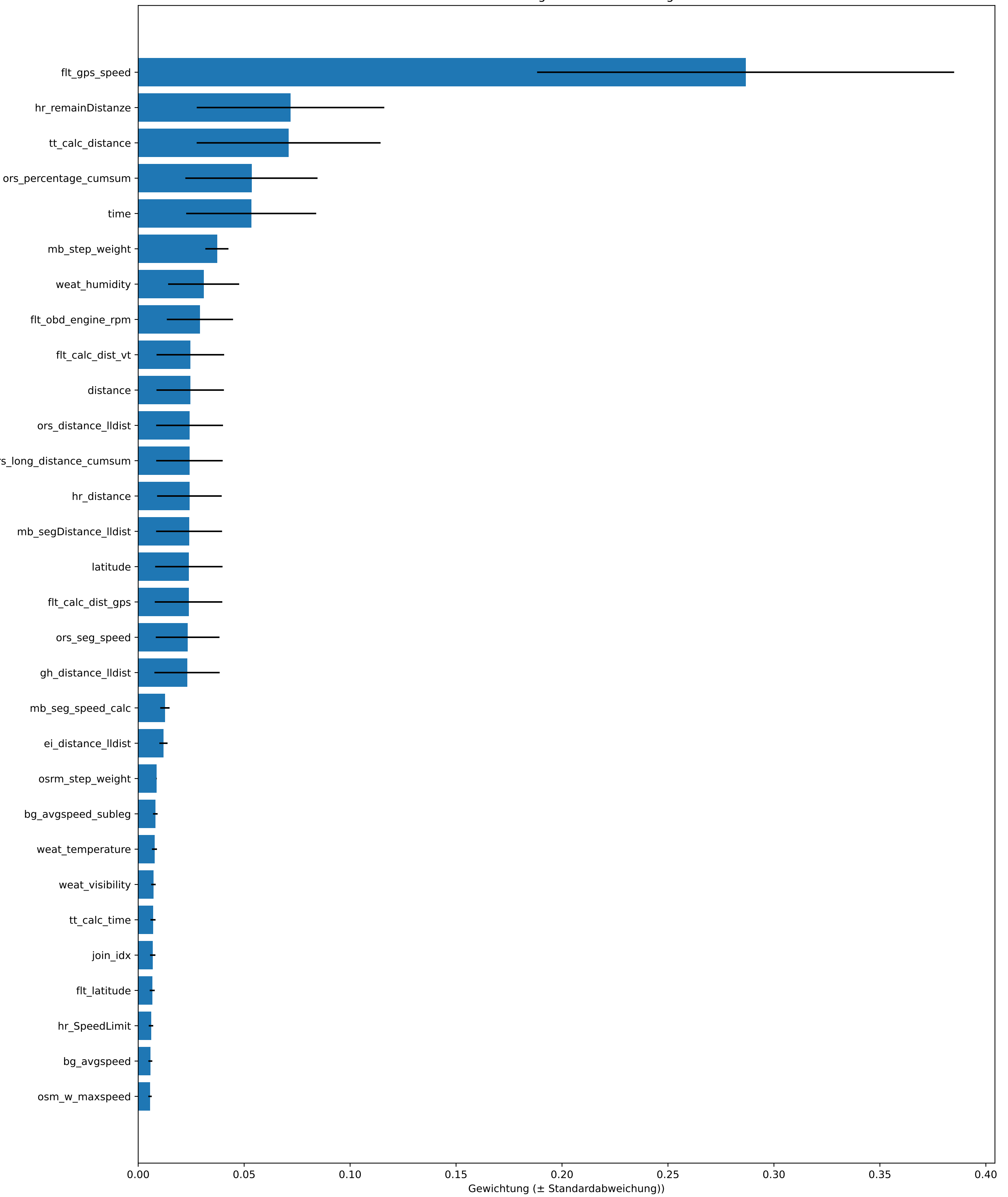
Feature-Gewichtung eines ExtreTreesRegressor
